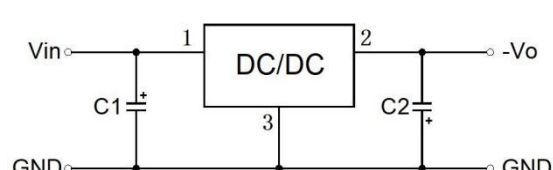
(图2) 负输出应用电路
