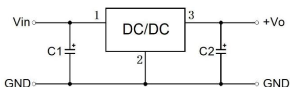
(图1) 正输出应用电路
